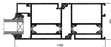
coupe de porte MB-60
