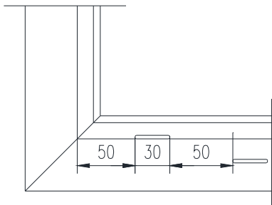
A chaque extrémité du dormant
