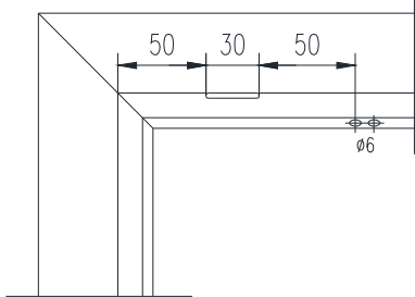
A chaque extrémité du dormant
