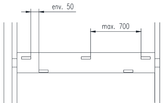
Traverse horizontale d'ouvrant
