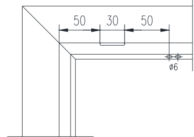
A chaque extrémité du dormant
