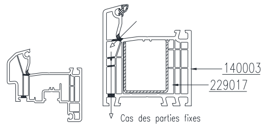
Cas des parties fixes
