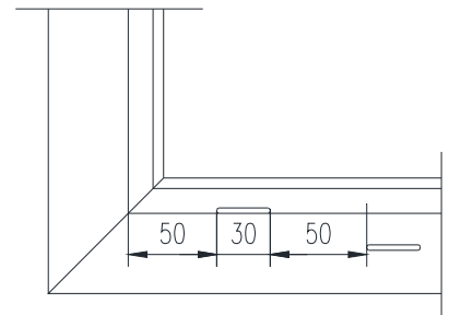
A chaque extrémité du dormant
