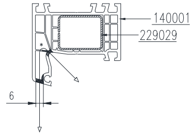
Cas des parties fixes
