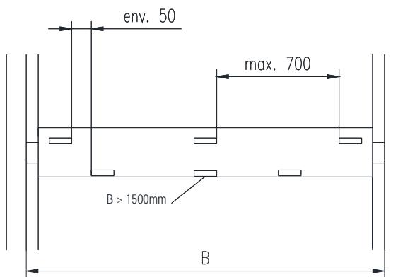
Meneau horizontal
